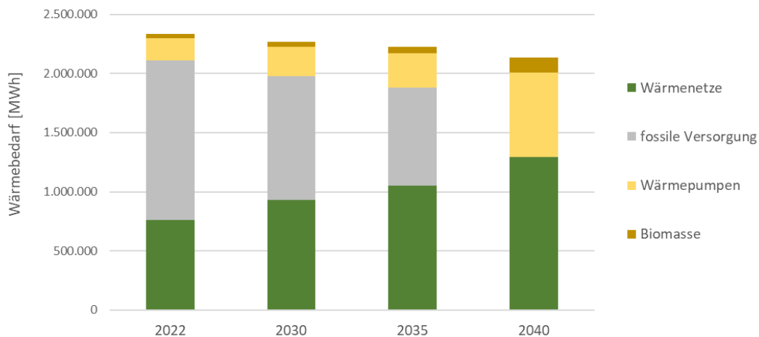
Abbildung 36: Entwicklung Endenergieträgereinsatz Wärme 2022 bis 2040 (Alternativszenario ohne Wasserstoff). Darstellung: GEF
