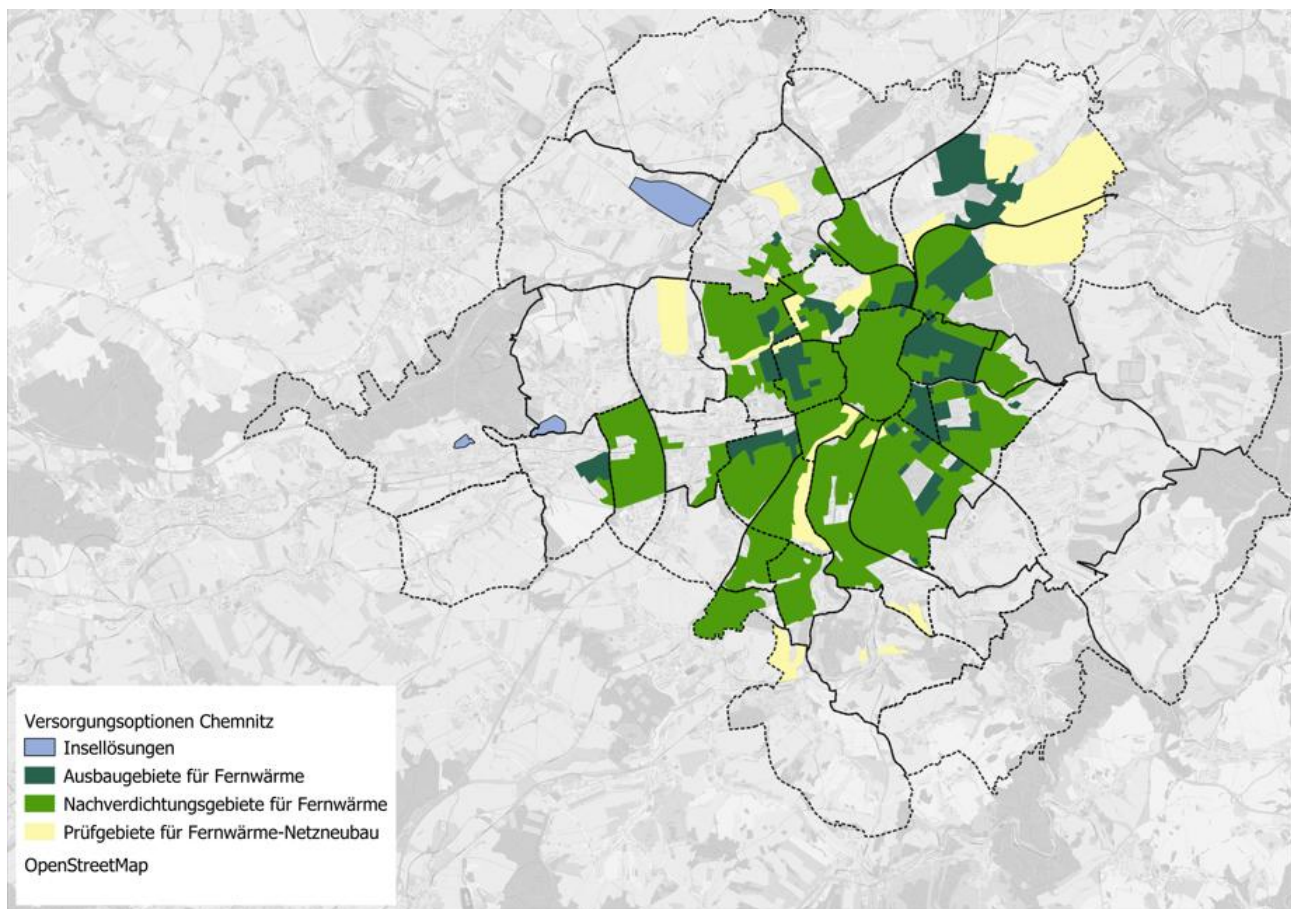
Abbildung 32: Eignungsgebiete für die Versorgung über ein Fernwärmenetz (Bestandsnetz, Netzausbau, Insellösungen und Prüfgebiete). Darstellung: GEF
