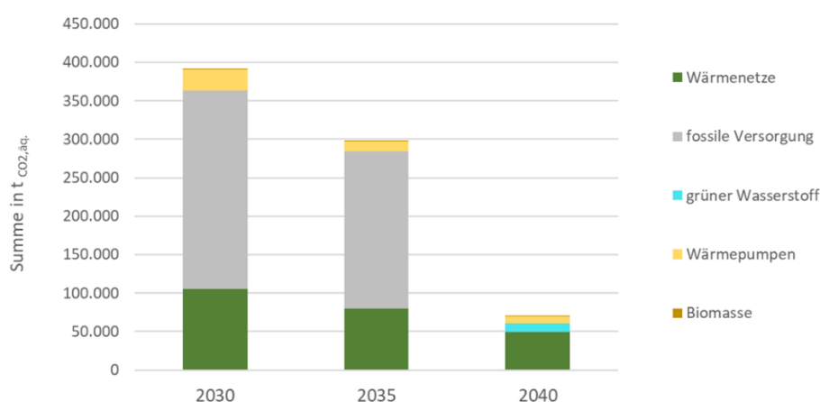
Abbildung 38: Entwicklung der THG-Emissionen im Zielszenario bis zum Zieljahr 2040. Darstellung: GEF
