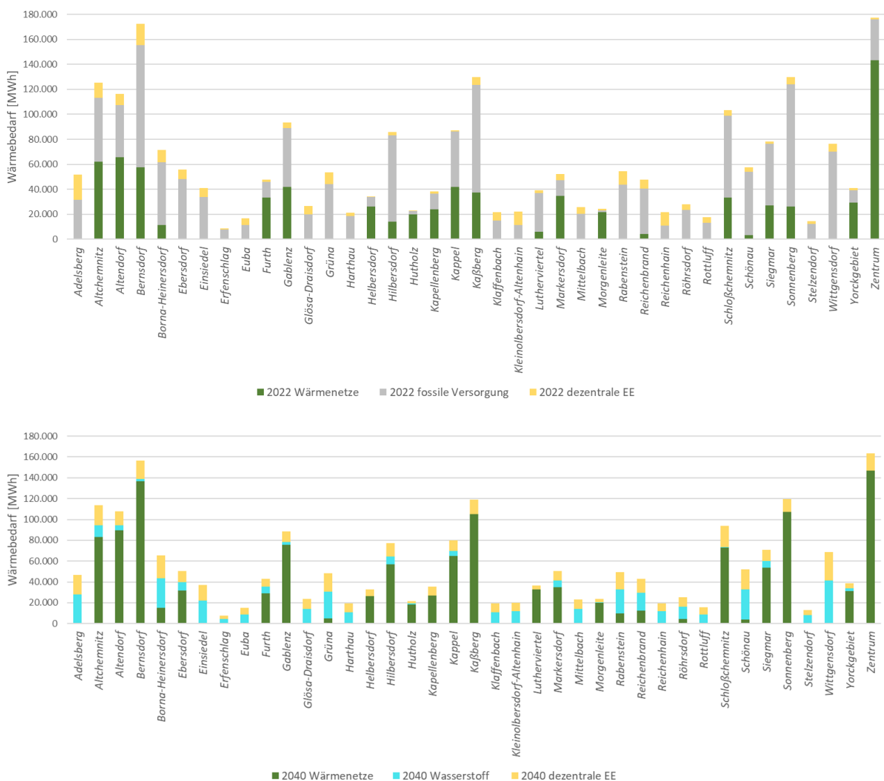
Abbildung 37: Stadtteilscharfe Darstellung der Wärmeversorgung nach Versorgungsoption; oben: Referenzjahr 2022, unten: Zieljahr 2040 . Aus Gründen der Darstellung erfolgt hier keine gesonderte Ausweisung der dezentralen EE-Energieträger (siehe Abbildung 35). Darstellung: GEF
